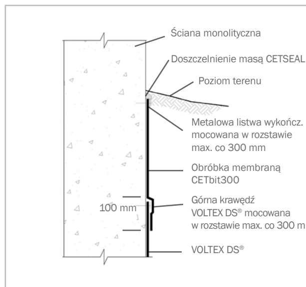
Zakończenie przy poziomie terenu
