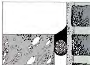
Rys. 1 Uszczelnienie przyfundamentowe
