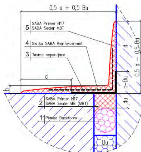
Wariant 3. Uszczelnienie narożnikowe
