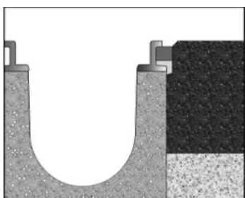
Szczegół 4. Uszczelnienie odwodnienia liniowego
