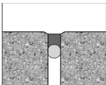
Szczegół 1. Dylatacja w betonie SABA Sealer na piance
