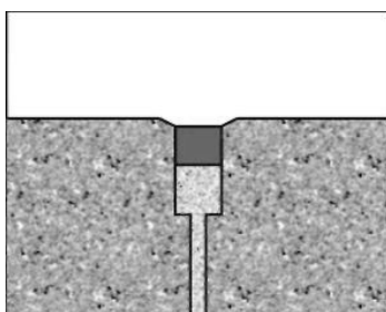
Szczegół 3. Dylatacja skurczowa SABA Sealer na piance
