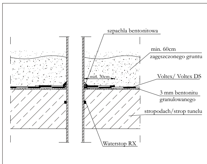
Rys. 43 - Szczegóły przejścia przewodu instalacyjnego przez stropodach przykrywany gruntem lub strop tunelu.
