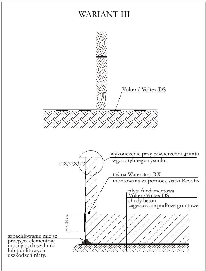
Rys. 11c - Sposoby przejścia izolacji poziomej na powierzchnię pionową. Wariant III.
