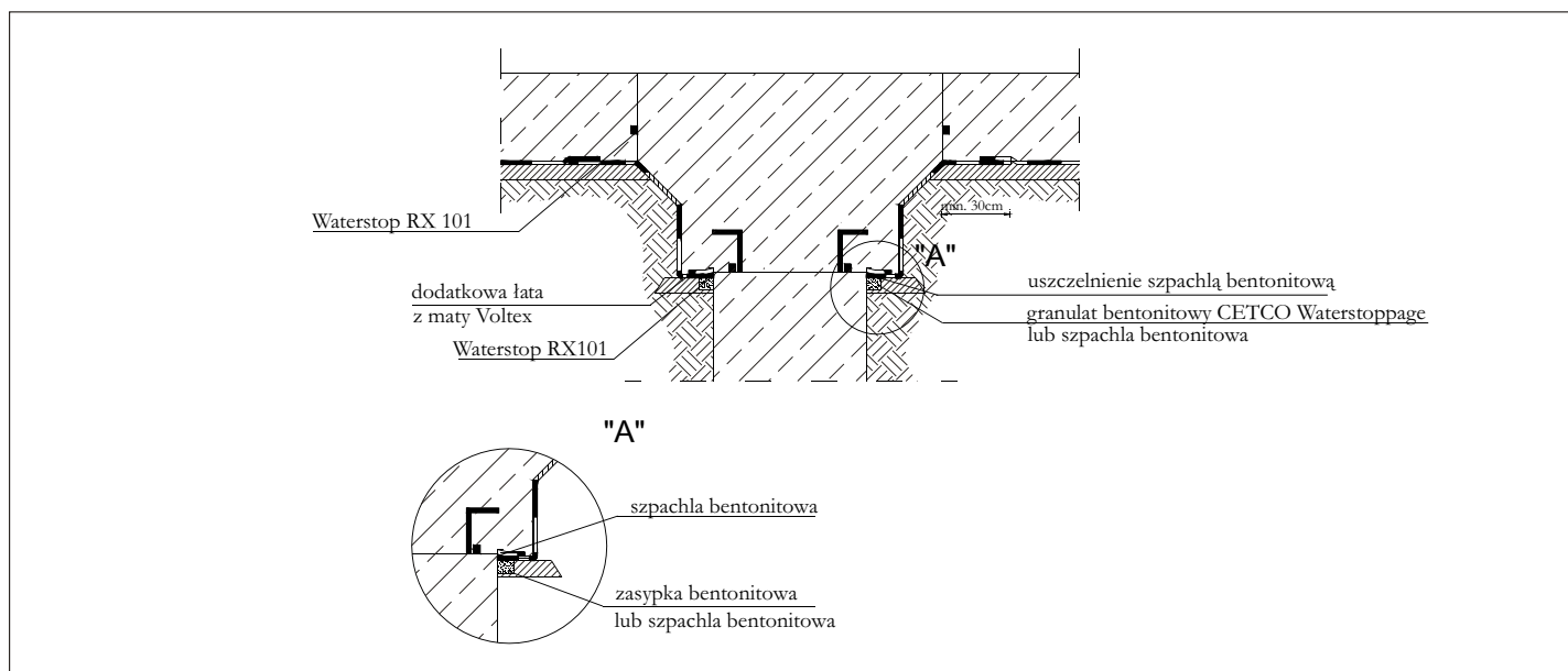
Rys. 6 - Szczegół izolowania oczepu pały.
