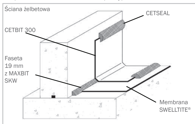
Stropodach – zakończenie membrany SWELLTITE w narożniku stropodachu
