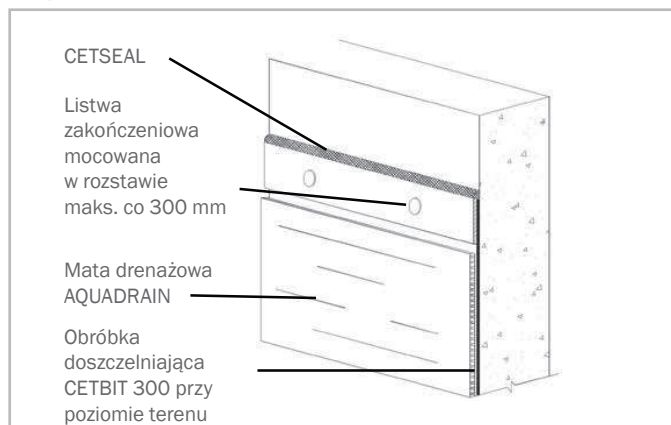
Typowe zakończenie przy poziomie terenu
