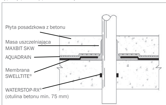
Przejście instalacyjne przez stropodach
