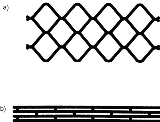
Rys. 1. Geokrata w pozycji rozłożonej i złożonej
