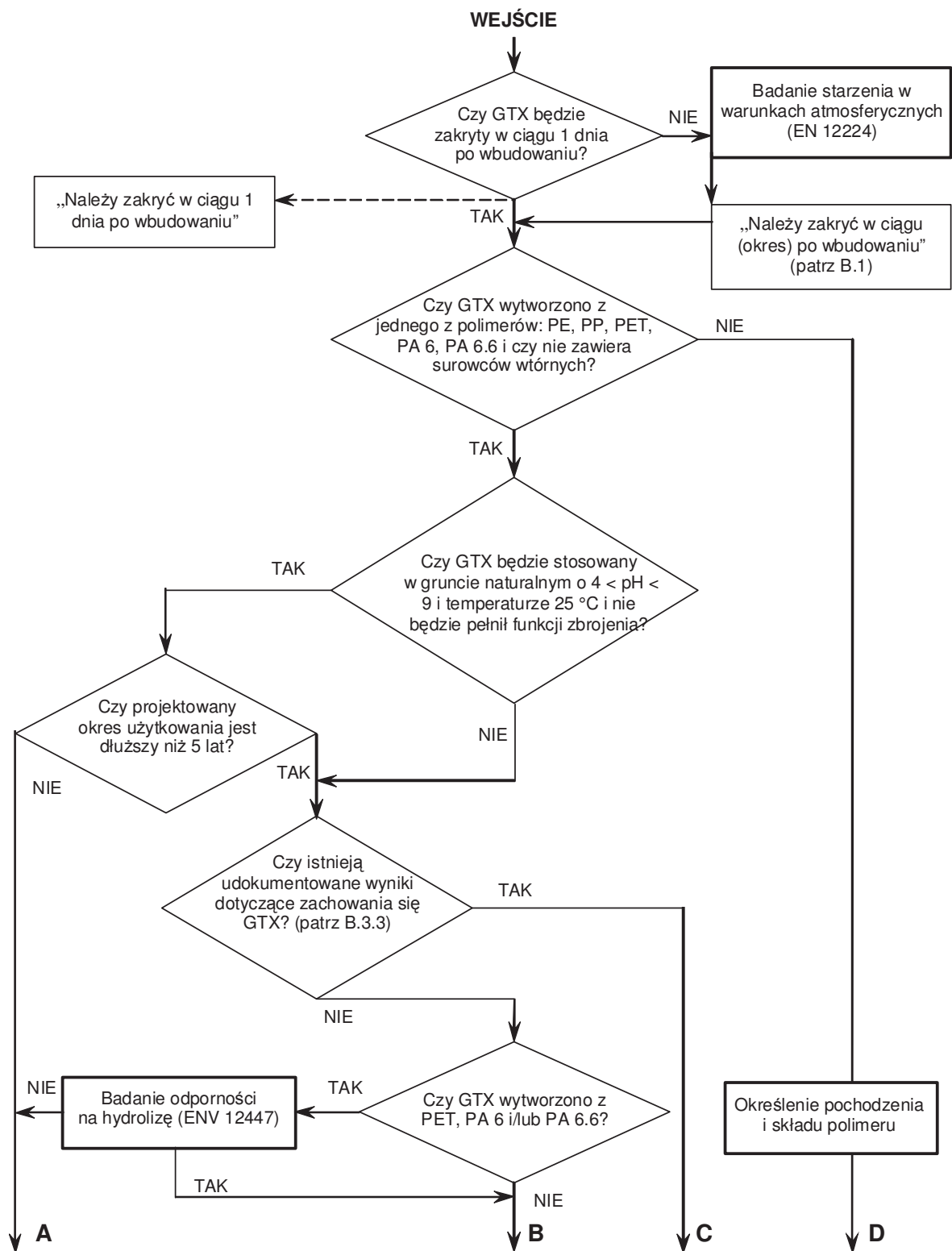
Rys. 9. Sposób oceny trwałości wg EN 13249
