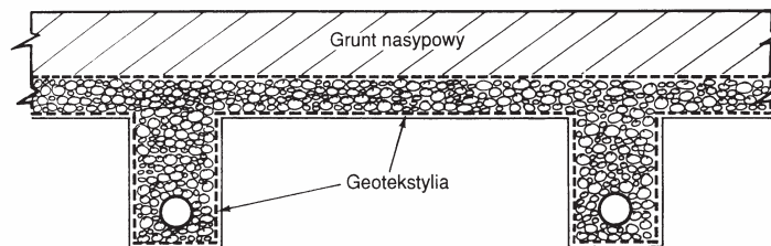
Rys. 19. Warstwa drenująca [29]
