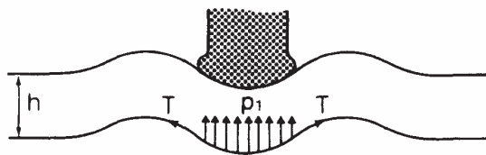
Rys. 27. Siła rozciągająca w zbrojeniu geotekstylnym [29]
