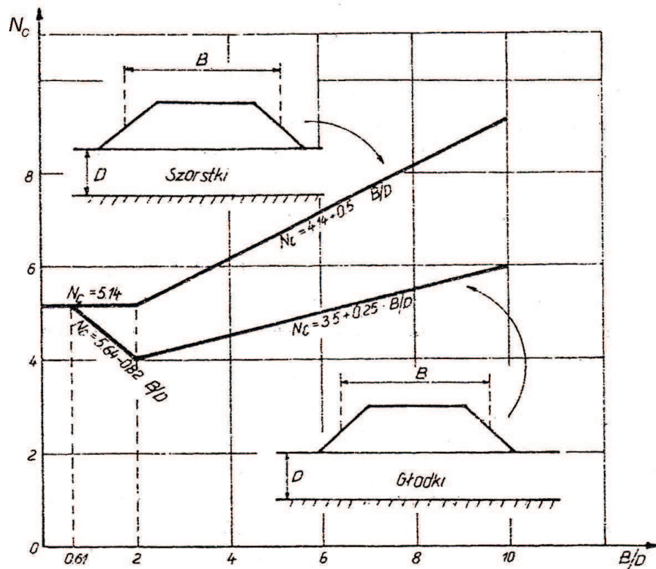
Rys. 36. Współczynnik nośności N_c do obliczenia nośności podłoża nasypu [27]
