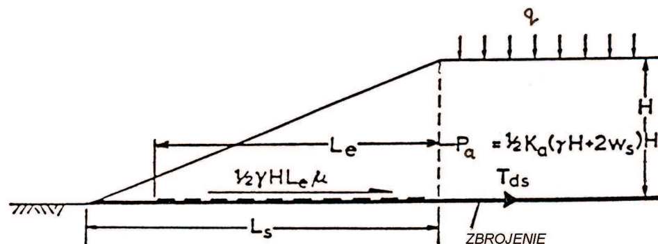
Rys. 34. Stateczność styku zbrojenia i nasypu
