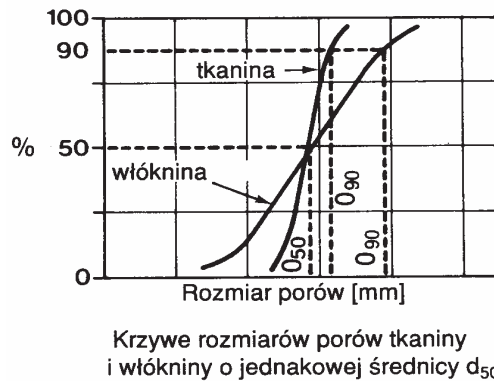
Rys. 21. Krzywe rozmiarów porów tkaniny i włókniny o jednakowej średnicy d_{50} [29]
