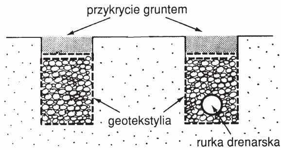
Rys. 18 Drenaż poziomy [29]
