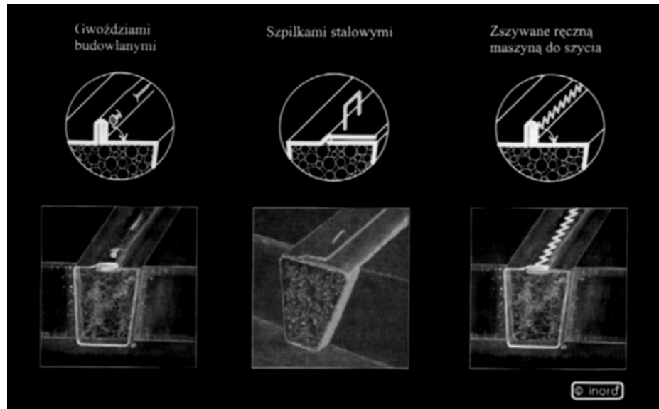
Rys. 25. Przykładowe sposoby zamykania drenu francuskiego [25]
