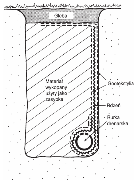
Rys. 20. Dren żebrowy [29]
