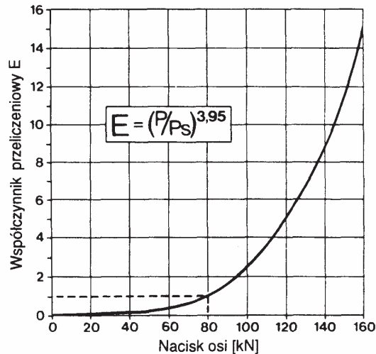
Rys. 28 Nomogram do przeliczenia obciążenia na osie standardowe
