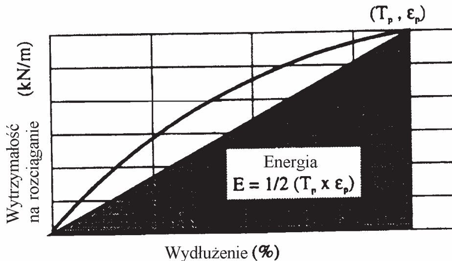
Rys. 8. Energia zniszczenia [57]
