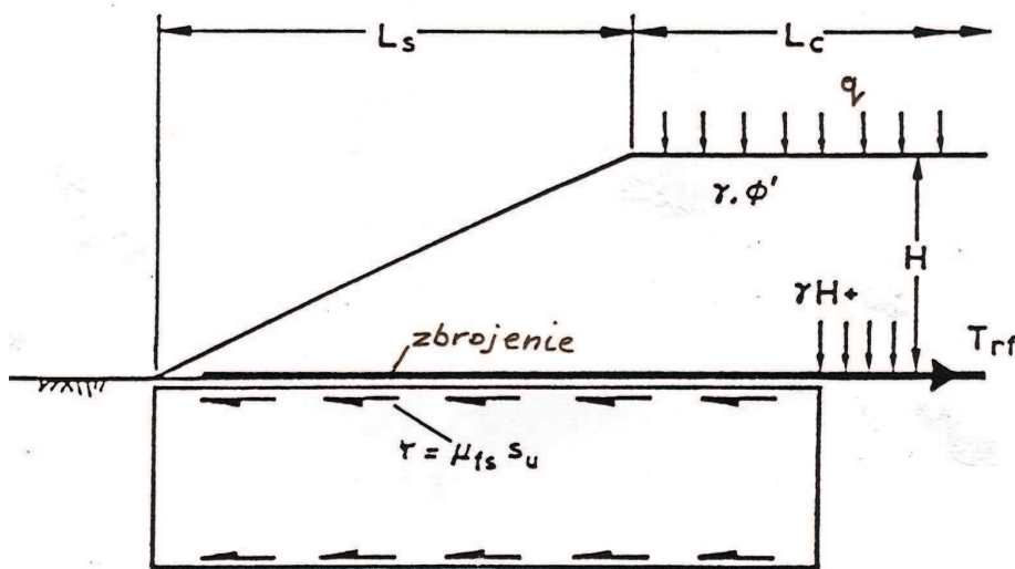
Rys. 35. Sprawdzenie możliwości wyparcia podłoża nasypu
