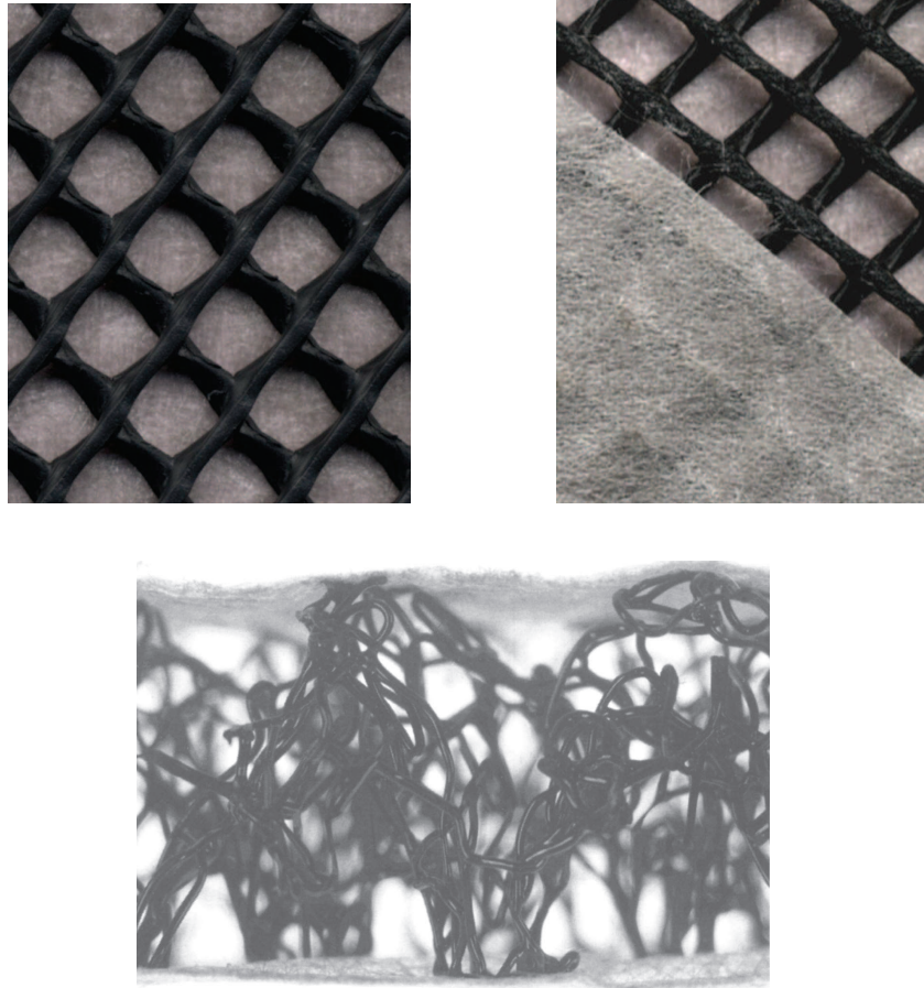
Rys. 4. Przykłady geokompozytów
