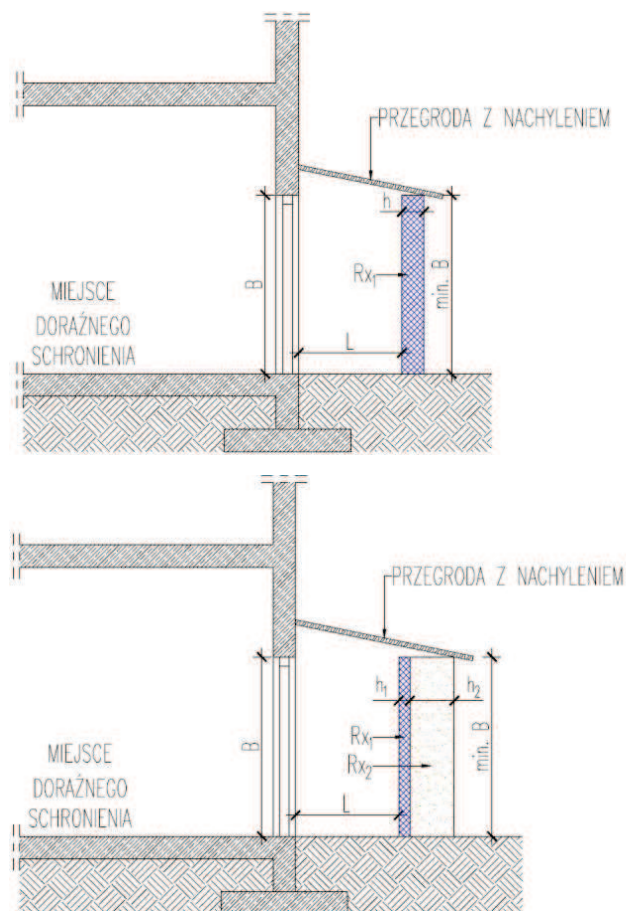
Rysunek 5. Przekrycie przestrzeni między ścianą zewnętrzną a osłoną okna lub wejścia do mds (przekrój).
