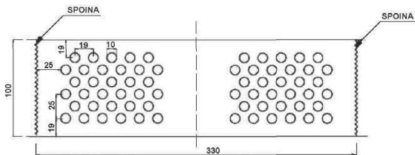
a) Perforacja taśmy o szerokości 100 mm, b) Perforacja taśmy o szerokości 200 mm
