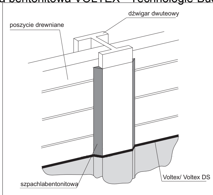
Rys. 30 - Sfazowanie szpachlą ostrego uskoku pomiędzy powierzchnią półki dźwigara i poszyciem drewnianym obudowy wykopu.
