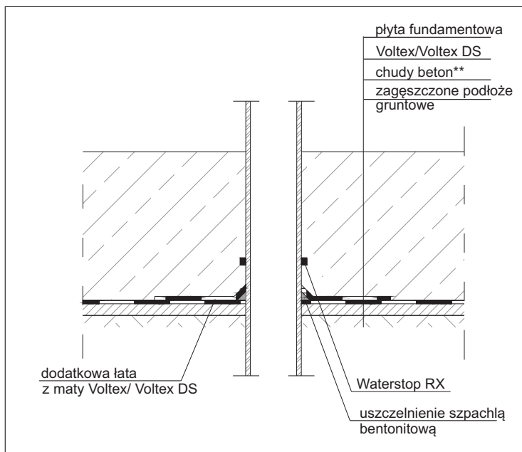
Rys. 8 - Uszczelnienie przejścia rury instalacyjnej przez płytę fundamentową.
