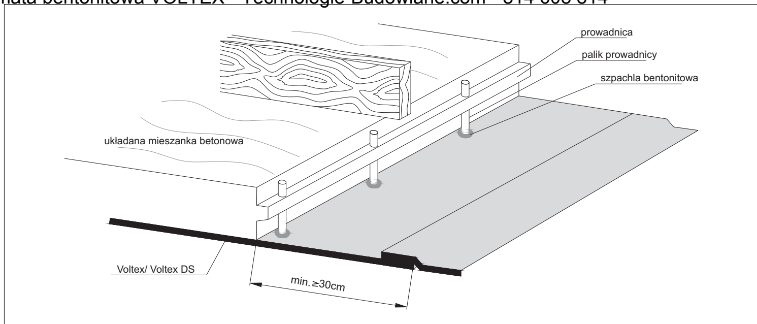
Rys. 18 - Przykład postępowania z palikami prowadnic.
