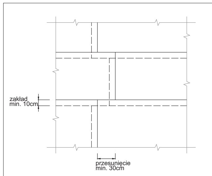
Rys. 3 - Schemat ułożenia maty pod płytą fundamentową.
