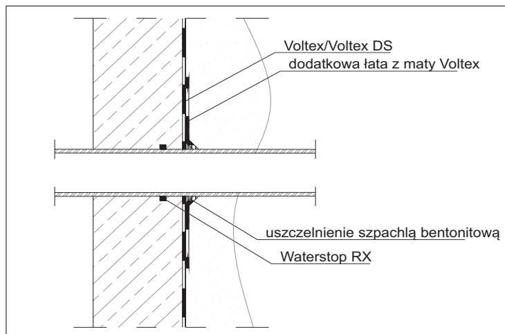
Rys. 24 Uszczelnienie przejścia rury instalacyjnej przez ścianę fundamentową.
