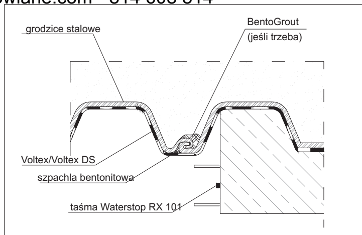
Rys. 38 - Szczegół uszczelnienia zamka grodzic stalowych - widok z góry.
