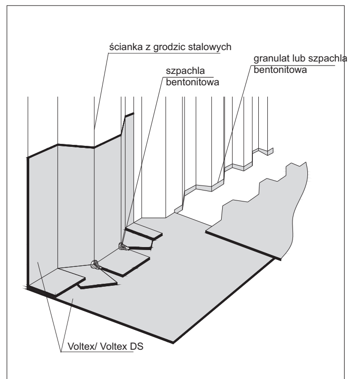
Rys. 17 - Połączenie izolacji poziomej z izolacją pionową układaną na grodzicach.
