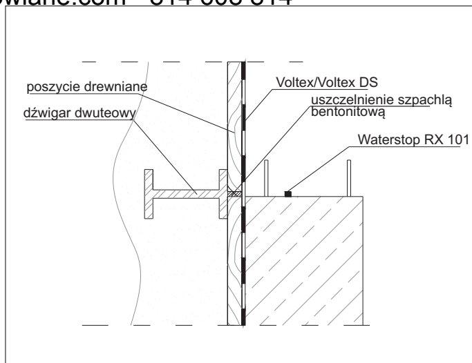
Rys. 33 - Bale obudowy na wewnętrznych półkach dźwigara - widok z góry.
