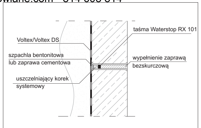
Rys. 21 - Szczegóły uszczelnienia w obrębie otworów po ściągach szalunków.
