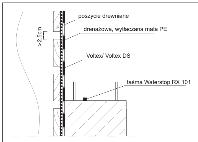
Rys. 32 - Drenażowa, wytłaczana mata PE użyta jako przykrycie nadmiernych przerw pomiędzy balami obudowy.
